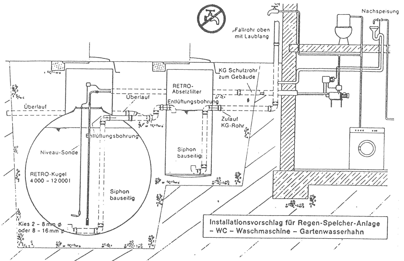
Regenwasserkugel Systemzeichnung Trockenversion mit Nachspeisung
